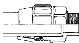
VISTA EN SECCIÓN DE UN ACCESORIO CORRECTAMENTE INSTALADO
